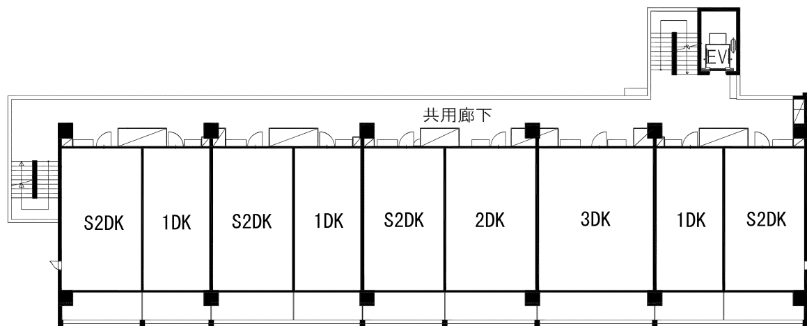
3～9階平面図
