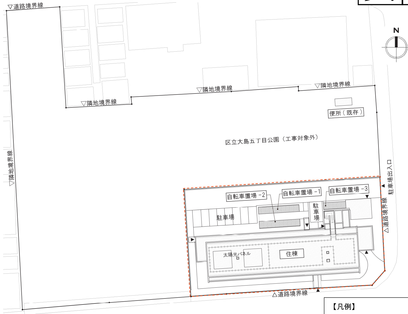
配置図
