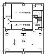
P3階
