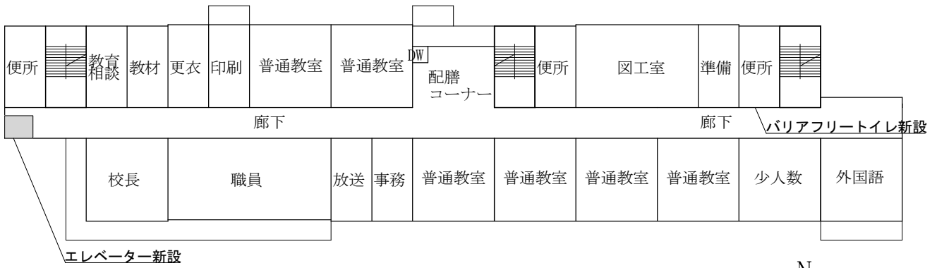
校舎棟 2階 S=1:500
