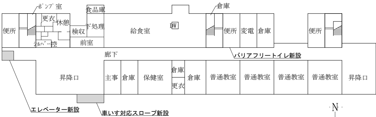
校舎棟 1階 S=1:500
