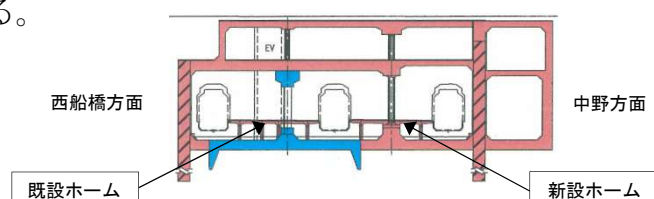
図3 完成形ホーム断面図
