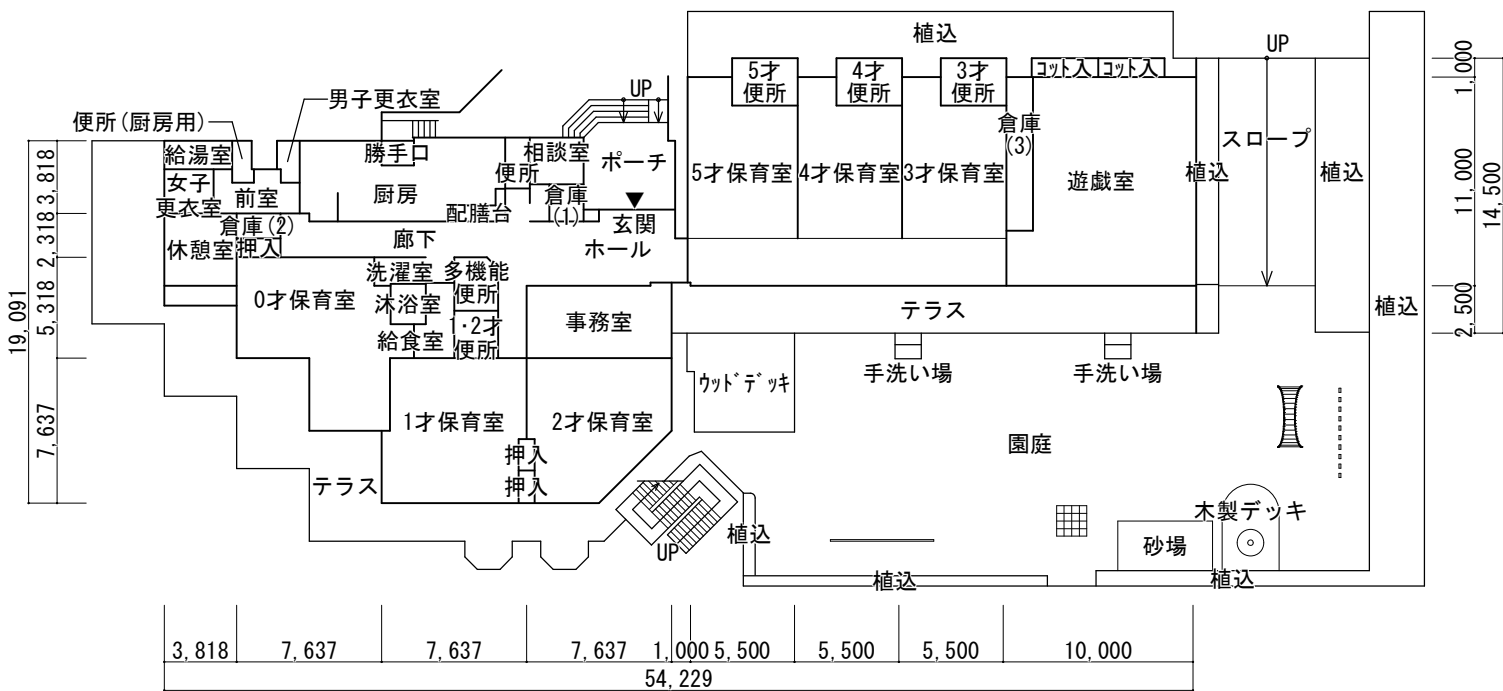
1階平面図 S=1:400
