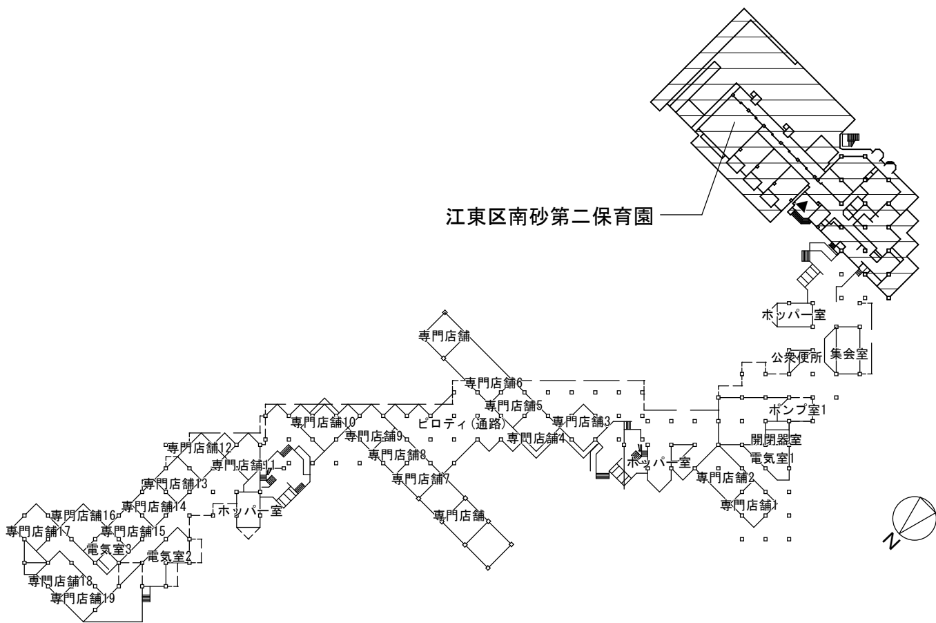
東京都住宅供給公社 南砂二丁目住宅1号棟 配置図 S=1:1200
