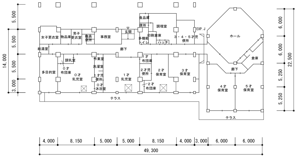
1階平面図 (改修後) S=1/400
