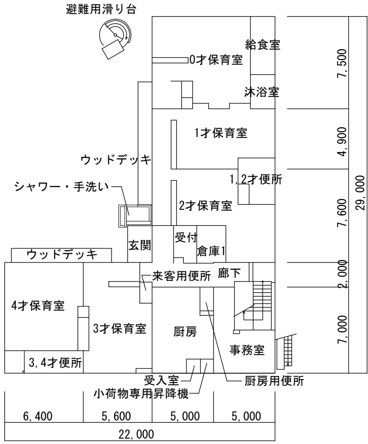
1階平面図 S=1:300 (A4)
