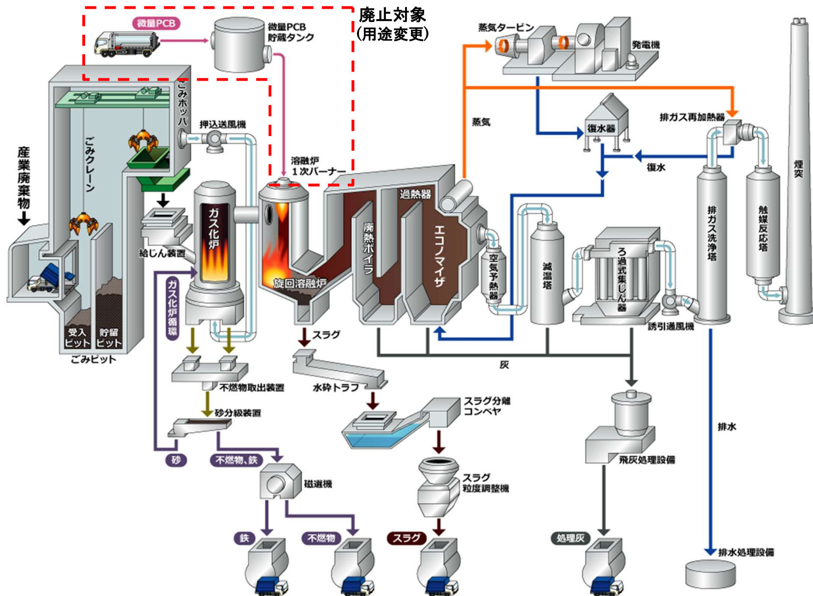
図 J & T 環境の産業廃棄物焼却及び微量PCB無害化の焼却設備
