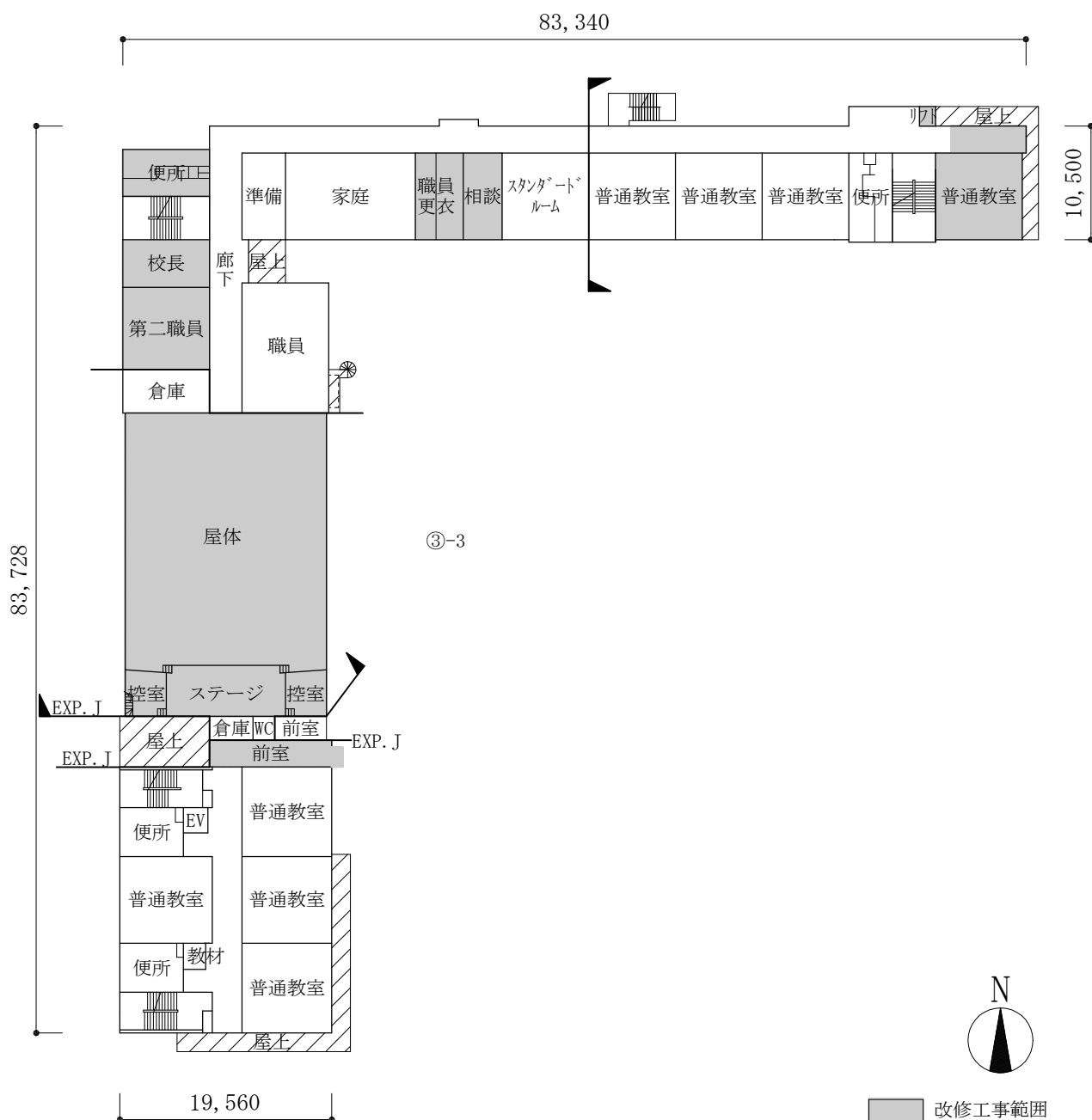
2階平面図 (改修後) SC=1:600
