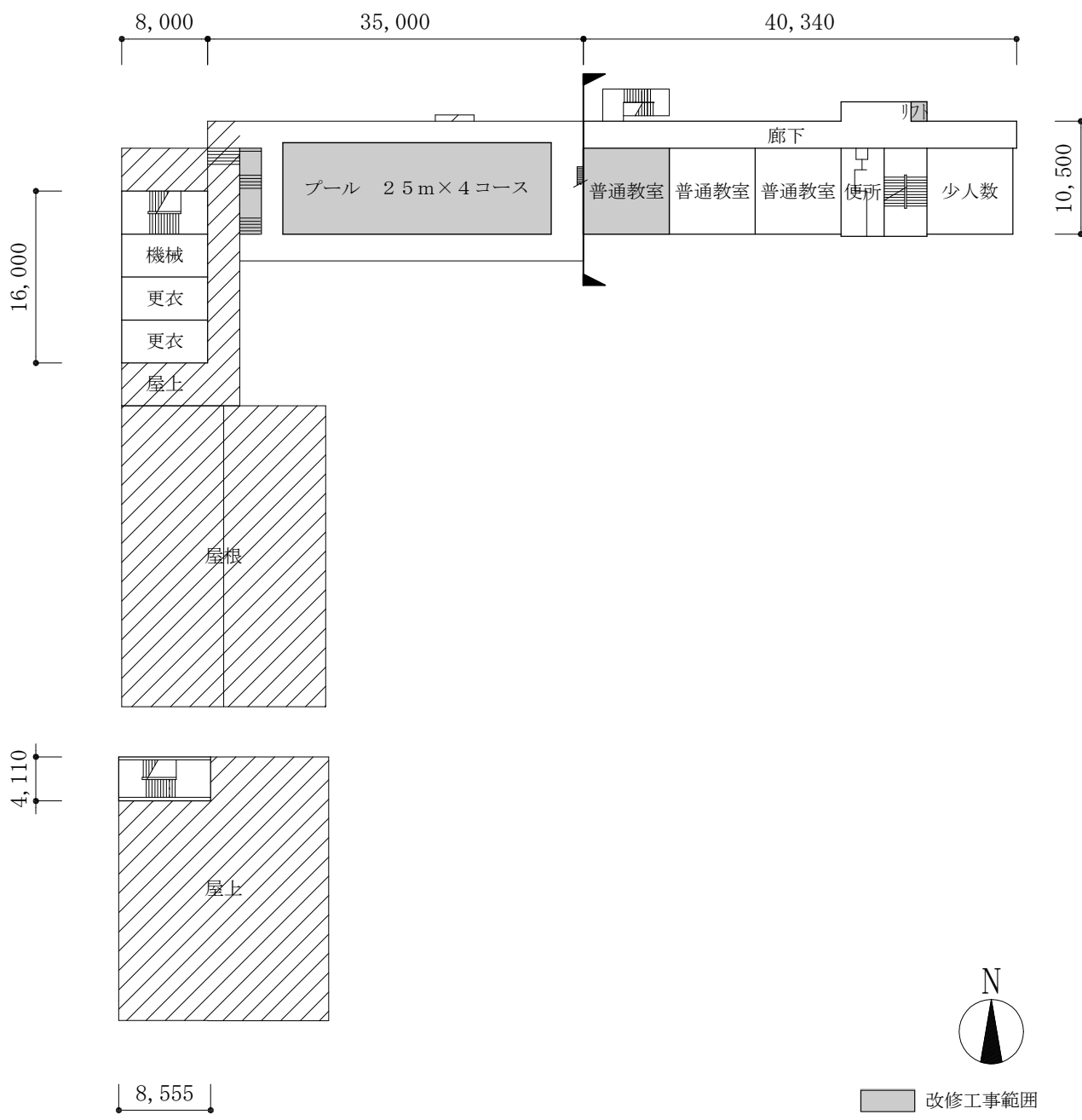
4階平面図 (改修後) SC=1:600
