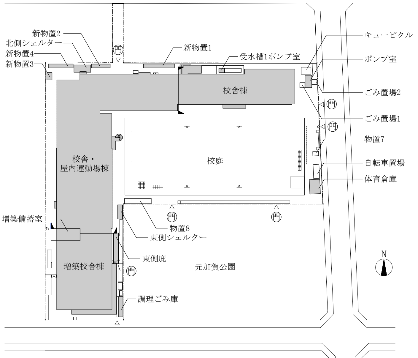
配置図 (改修後) SC=1:800
