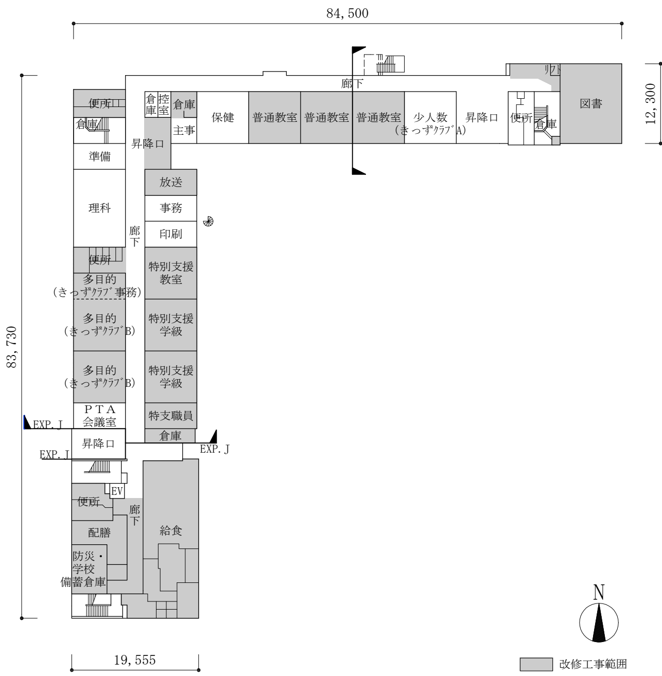
1階平面図 (改修後) SC=1:600
