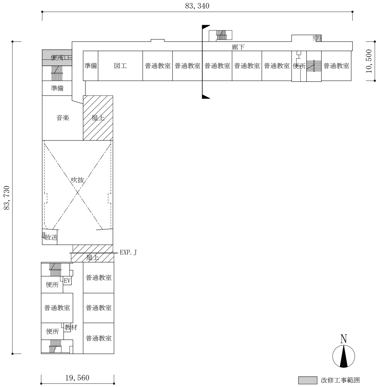
3階平面図（改修後）SC=1:600
