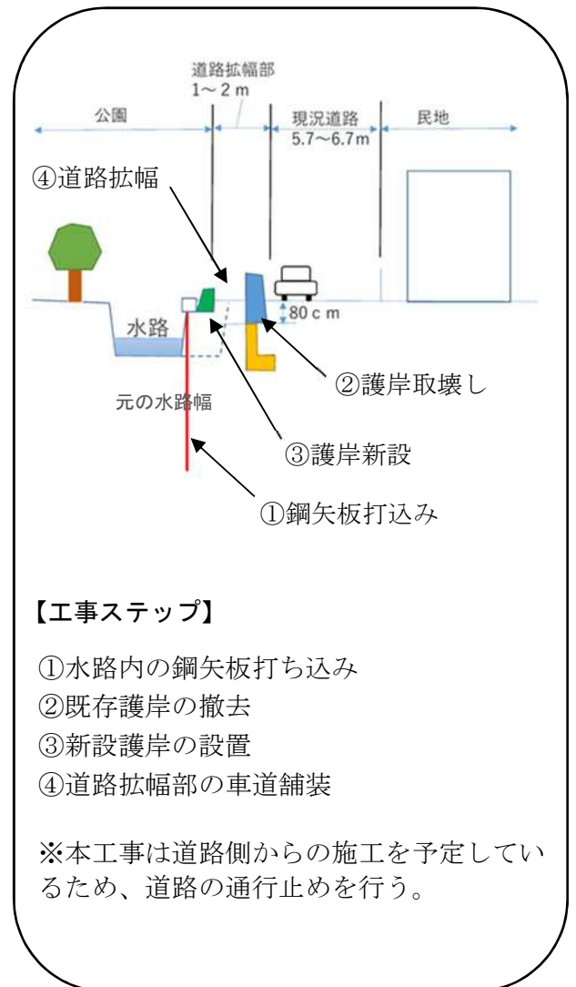
【標準断面図】
