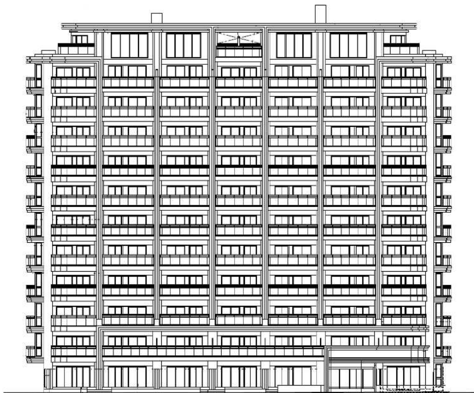
南側立面図
