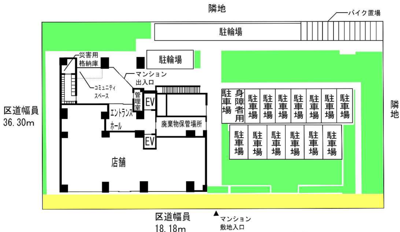
配置図
