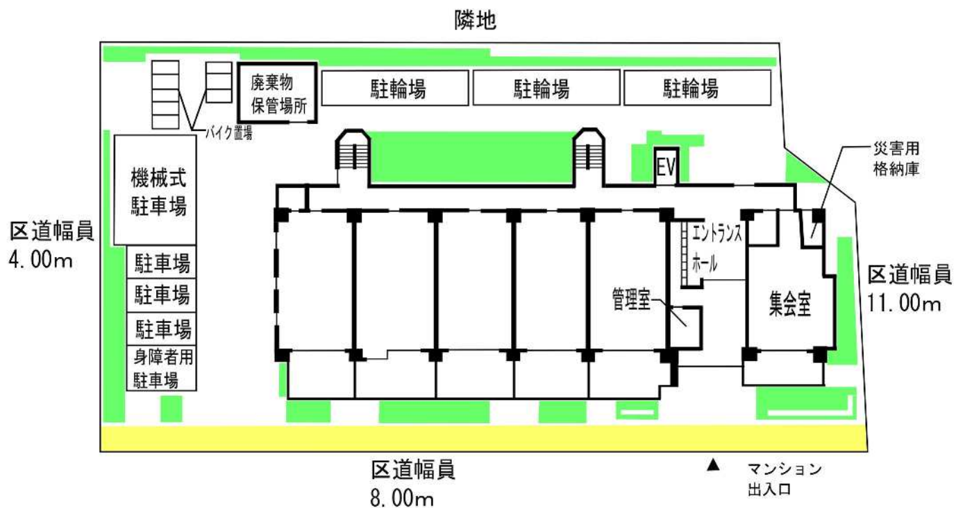
配置図
