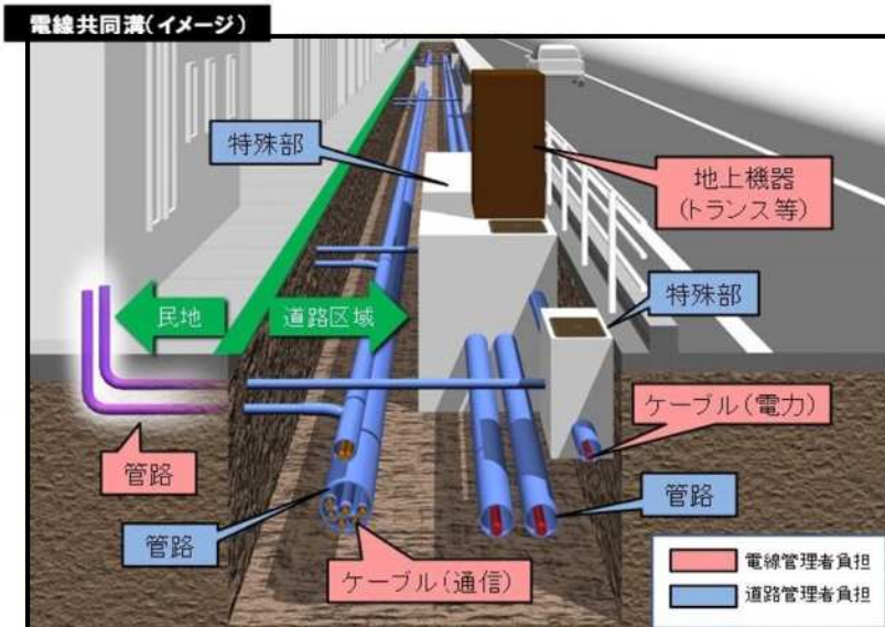
電線共同溝整備イメージ
