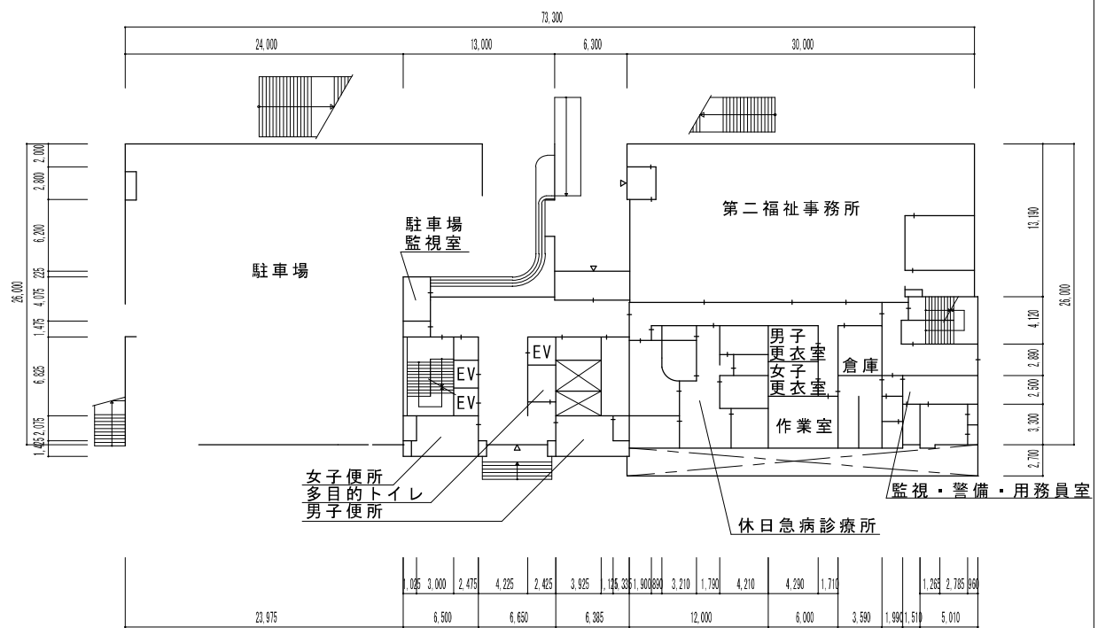
1階平面図 S=1/500
