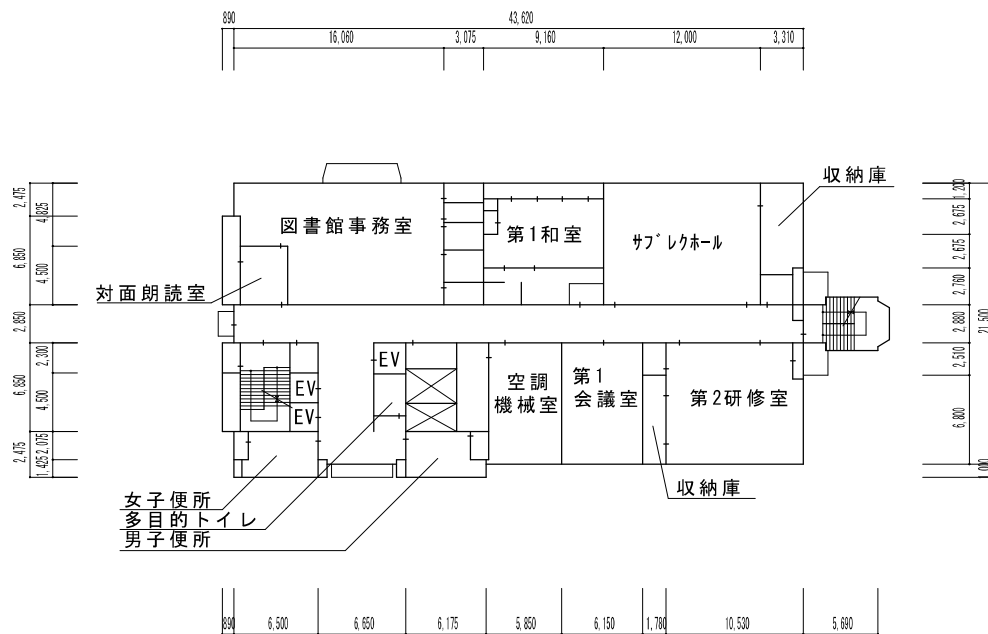
6階平面図 S=1/500
