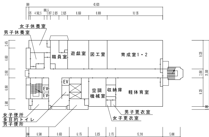
5階平面図 S=1/500
