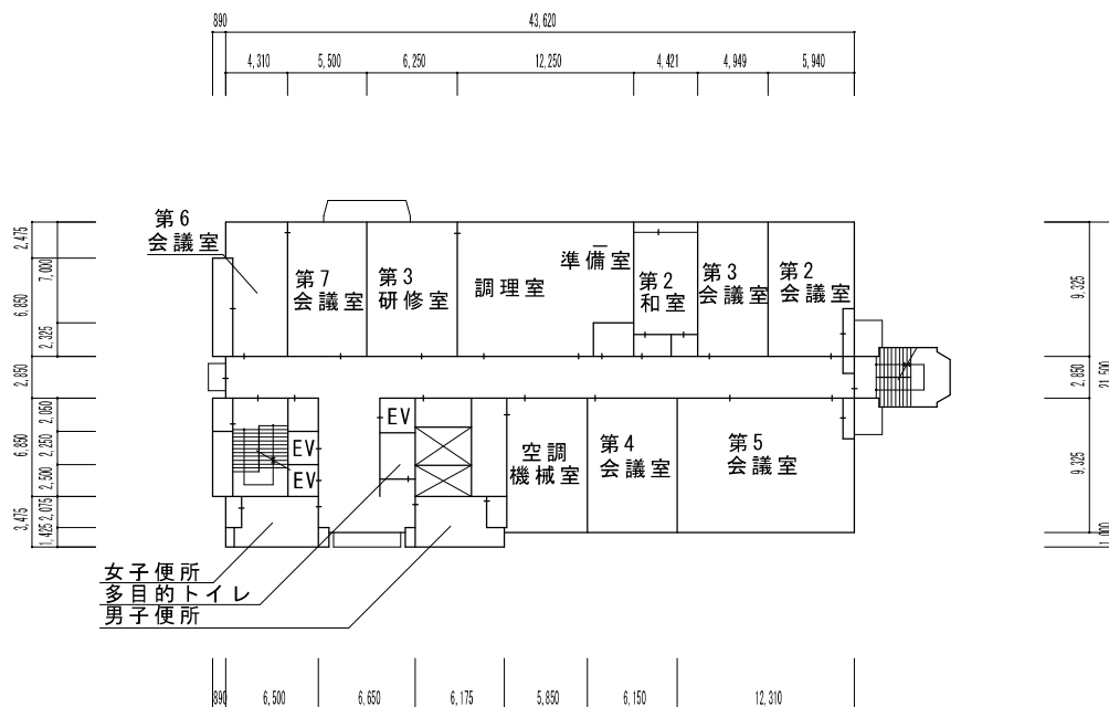
7階平面図 S=1/500
