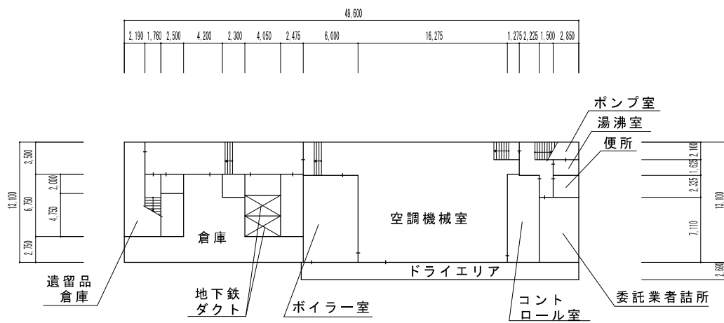
地下平面図 S=1/500
