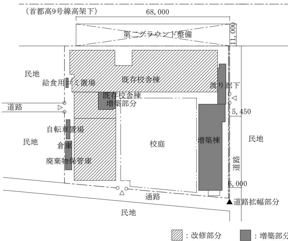
【配置図】 S = 1/1000
