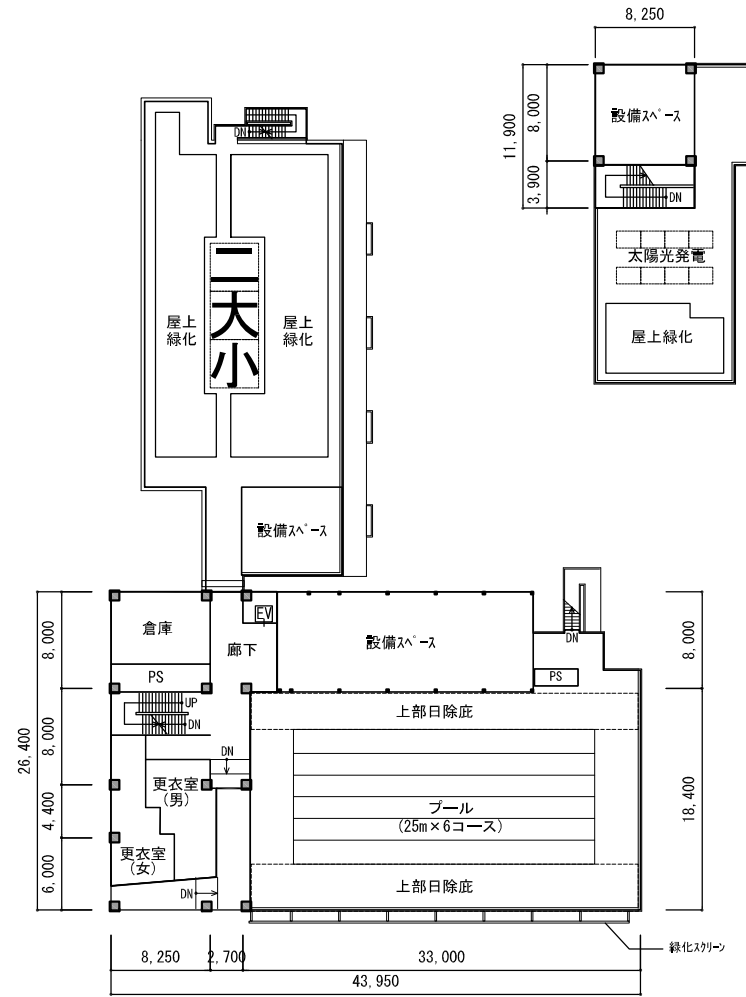
PH階平面図
