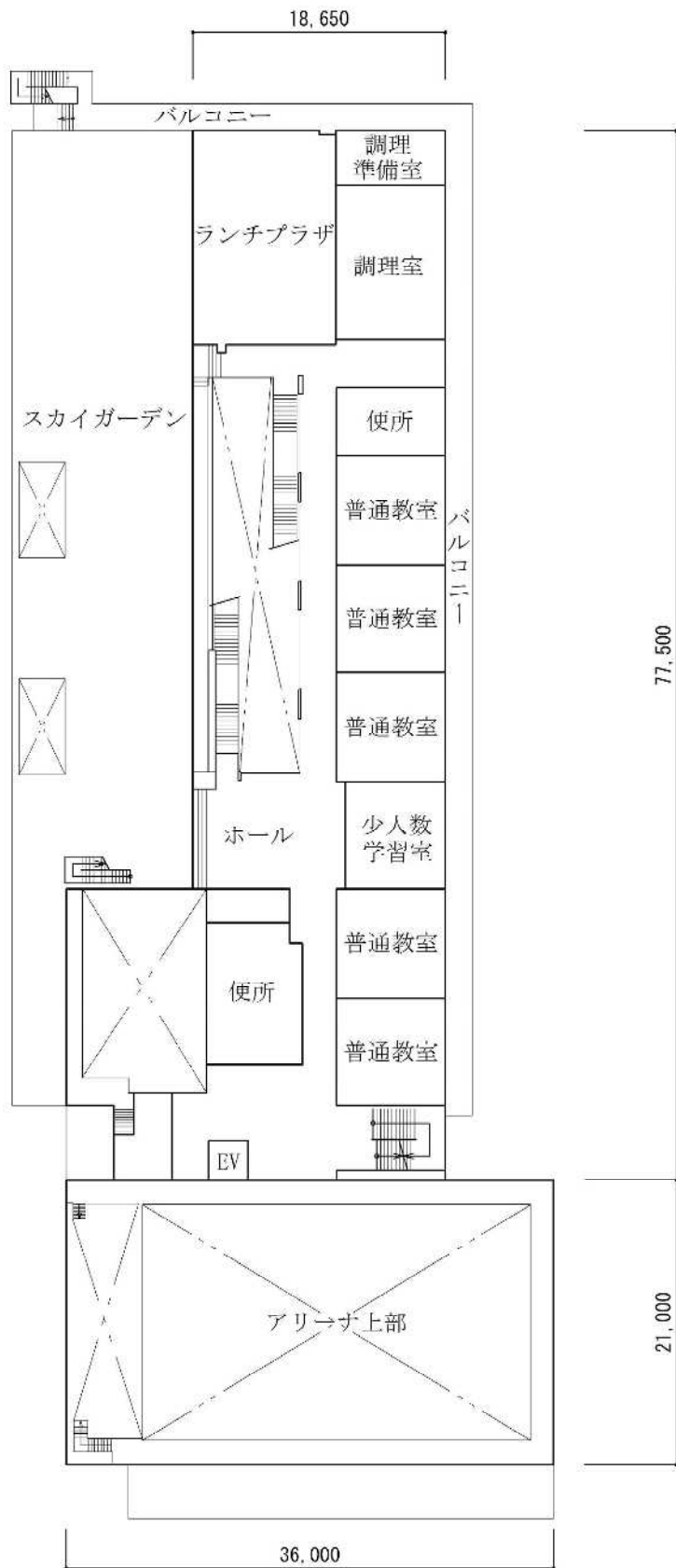
3階平面図
