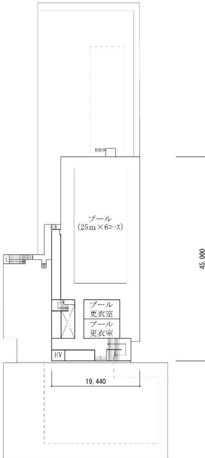
4階平面図
