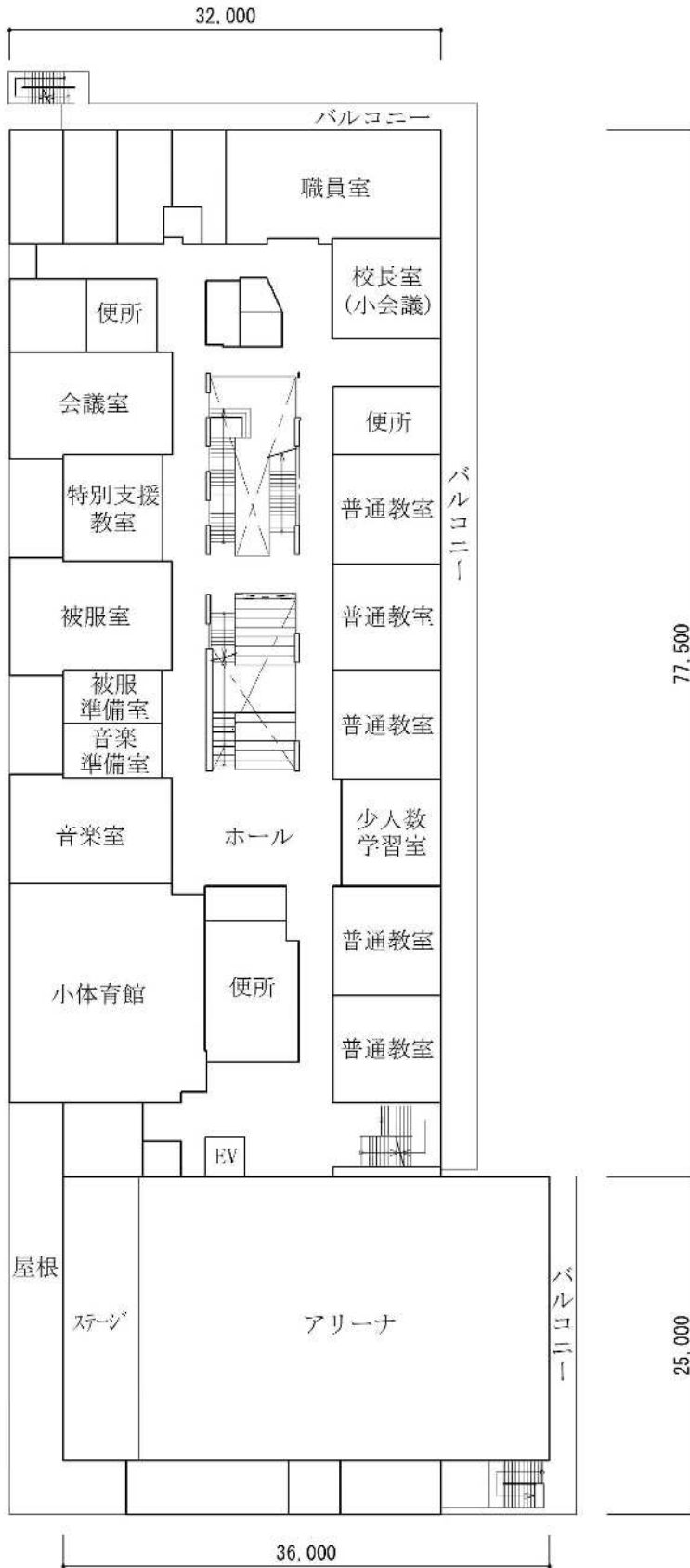
2階平面図
