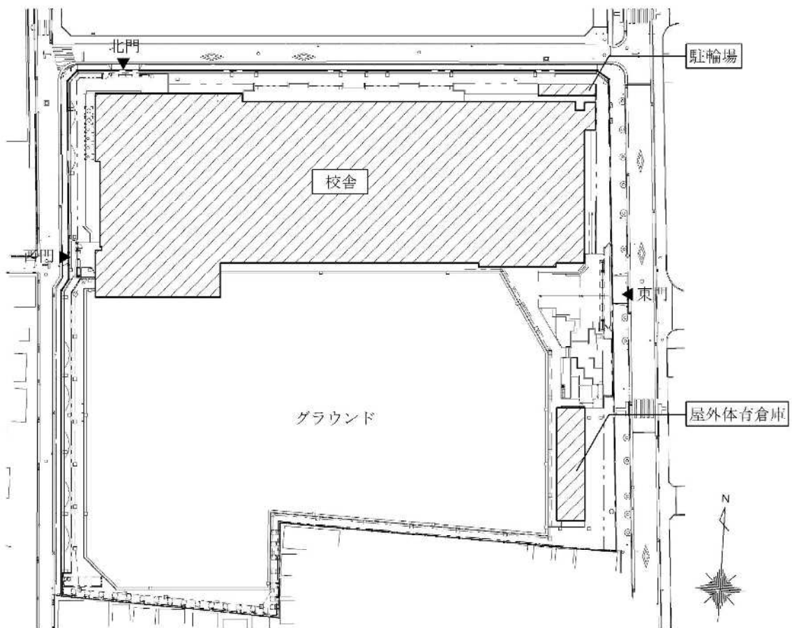
配置図
