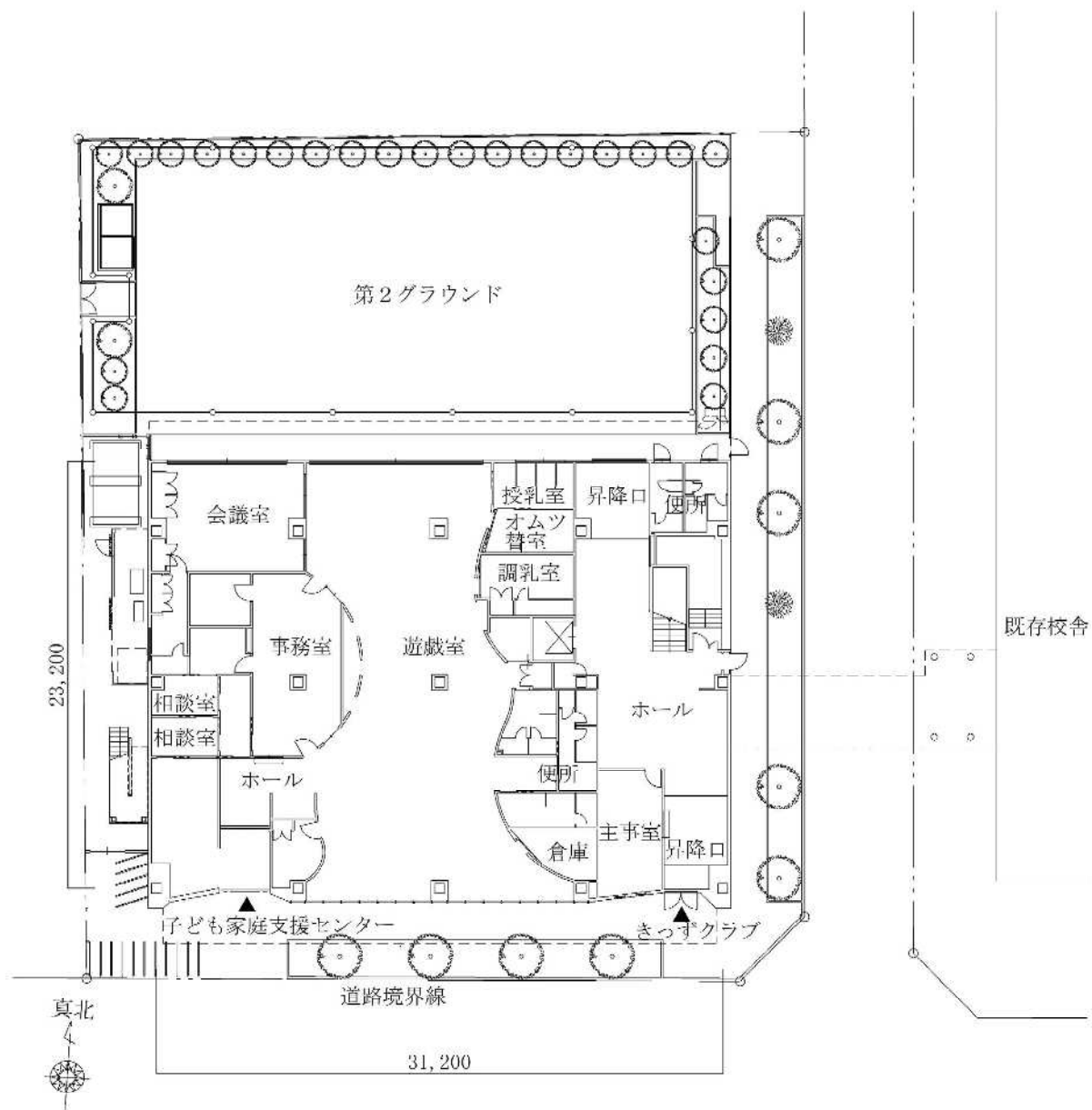
1階平面図
