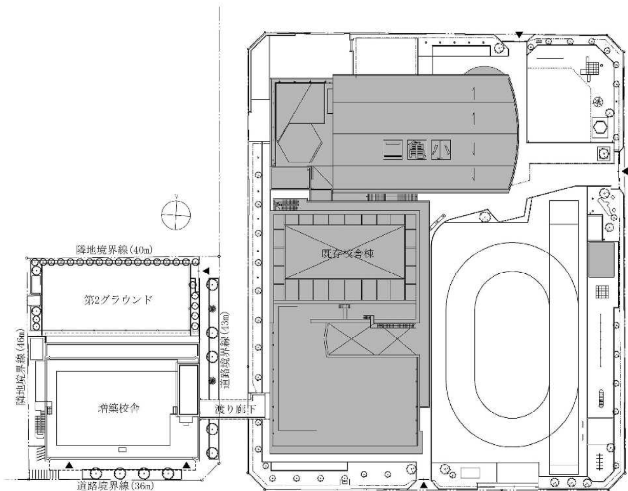
配置図
