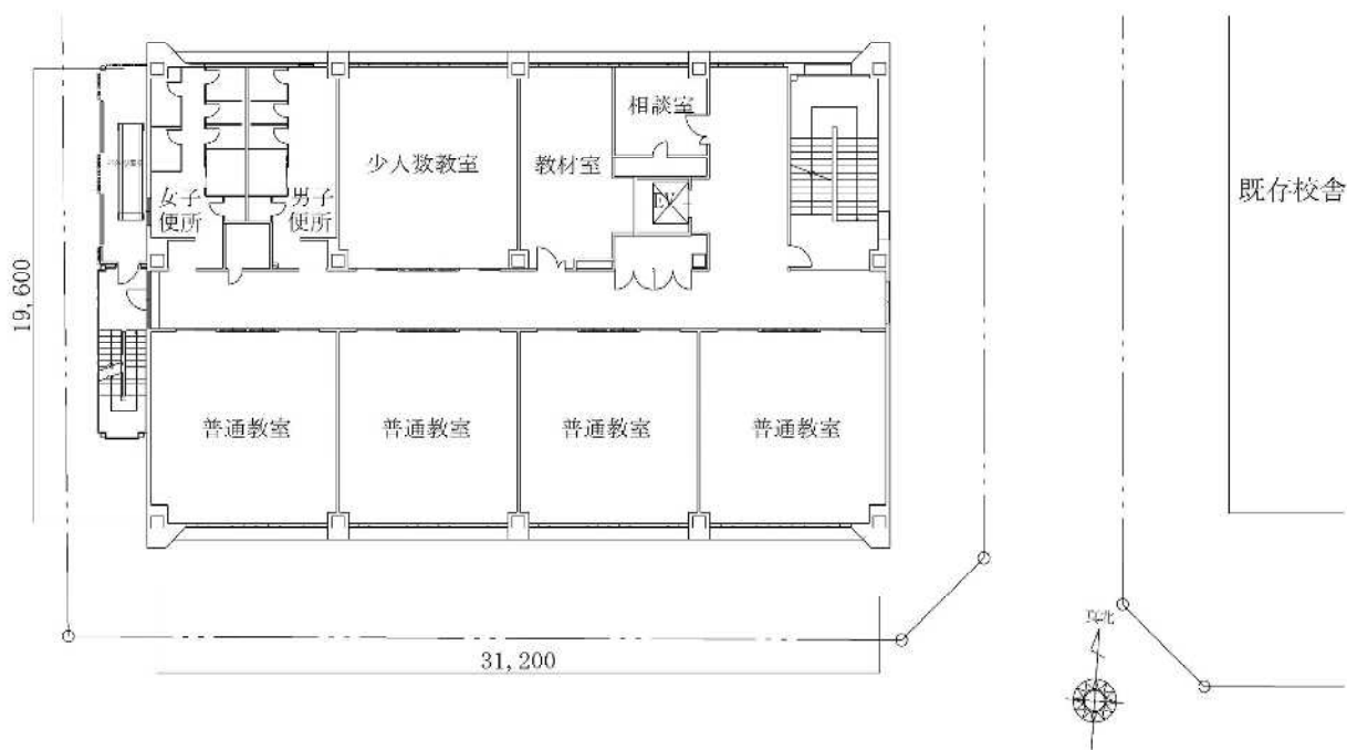
5階平面図
