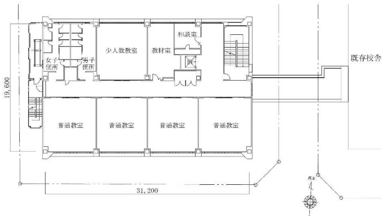
4階平面図
