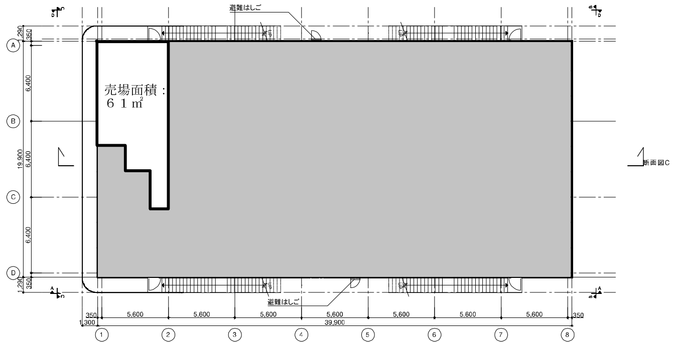
2階 平面図
