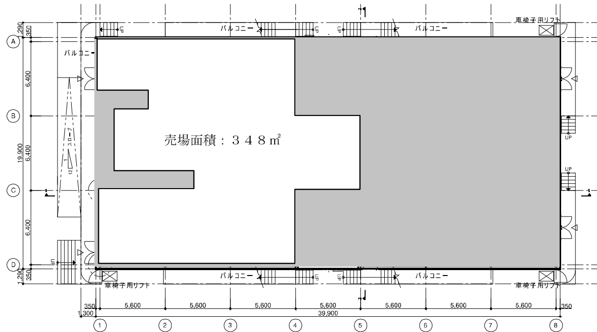
1階 平面図
