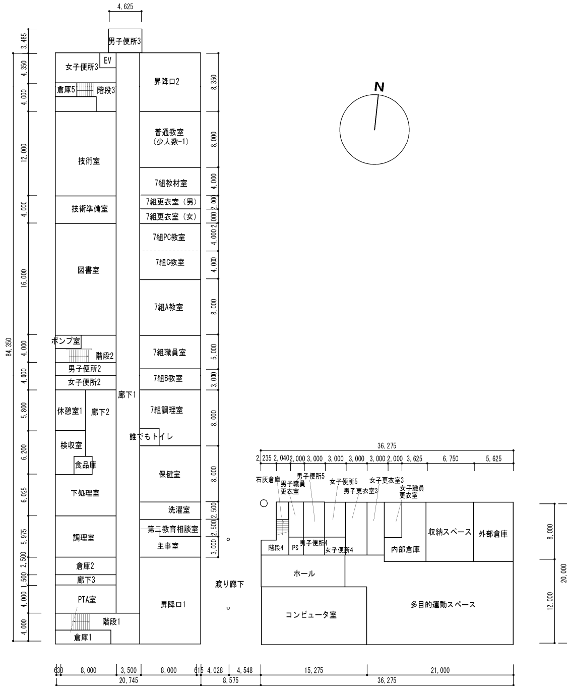
1階平面図 S=1/500
