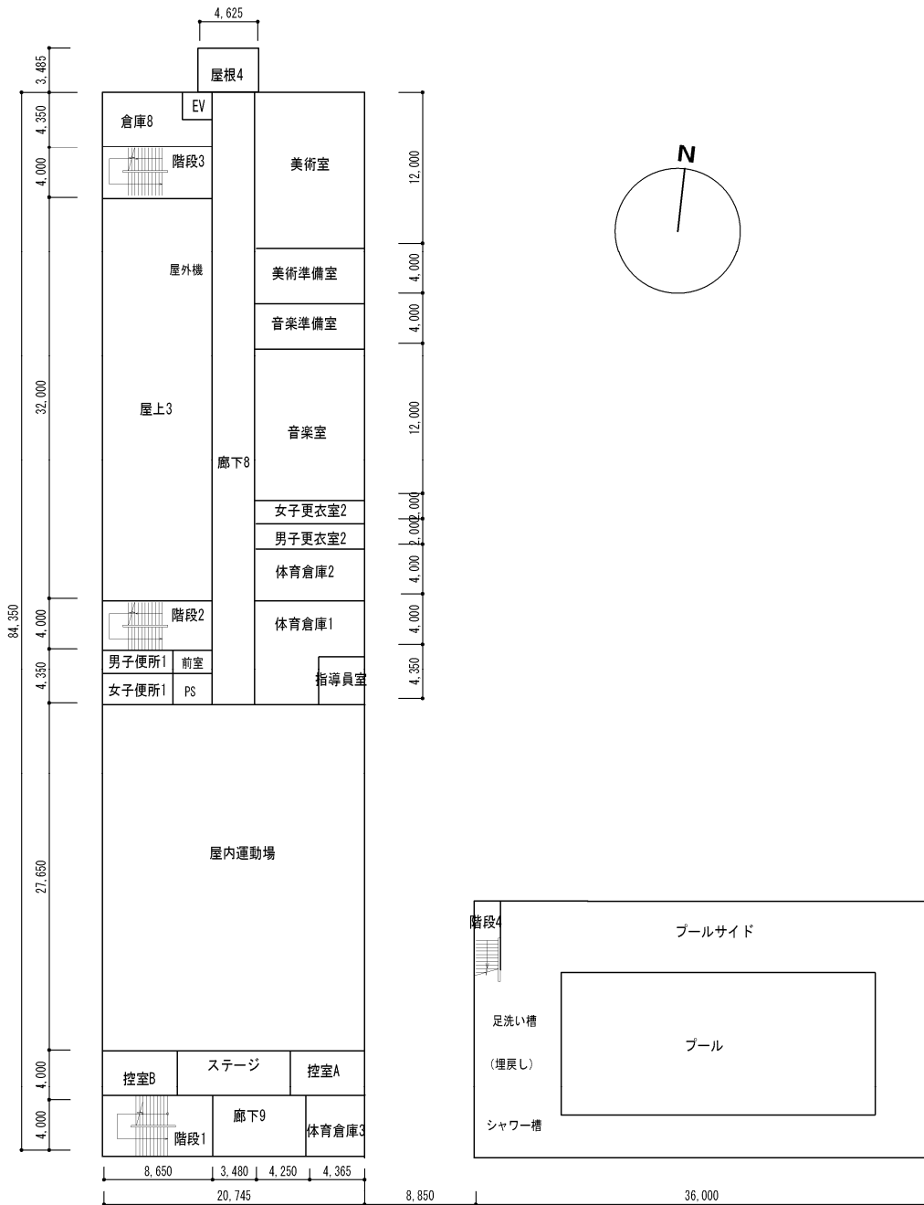
4階平面図 S=1/500
