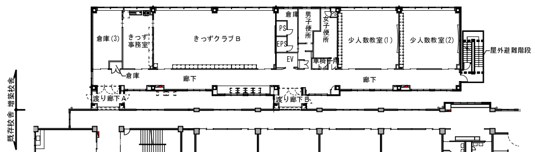
3階平面図 S=1/500
