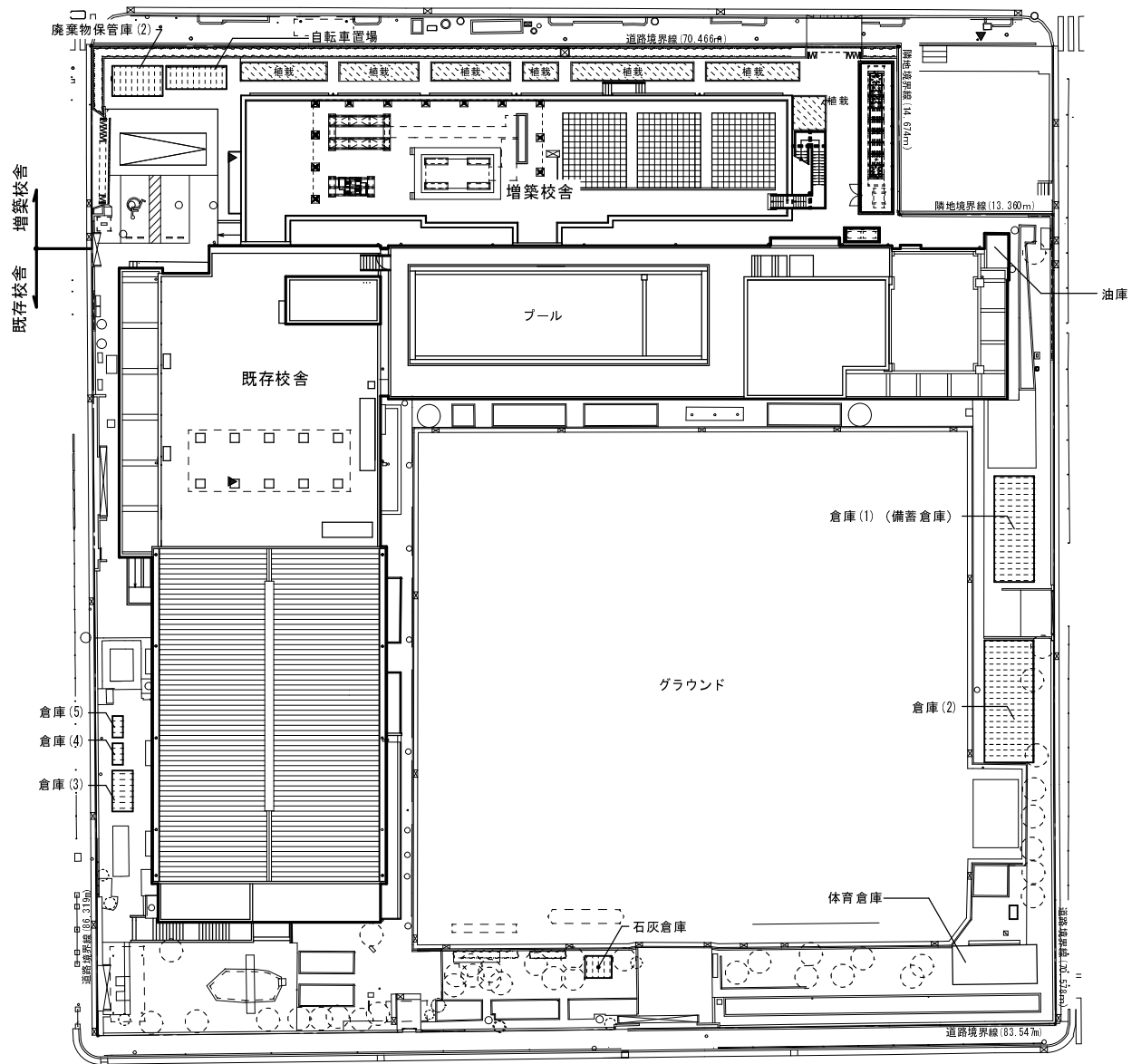
配置図 S=1/600
