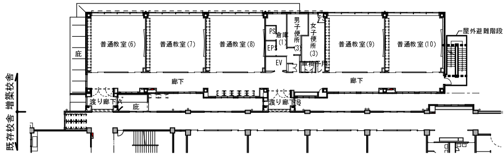
2階平面図 S=1/500
