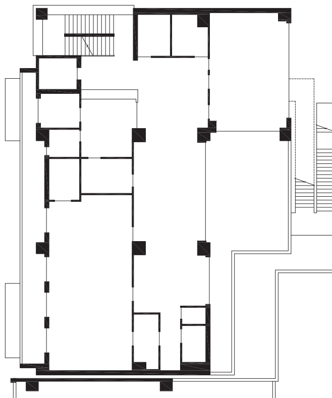
2階平面図
