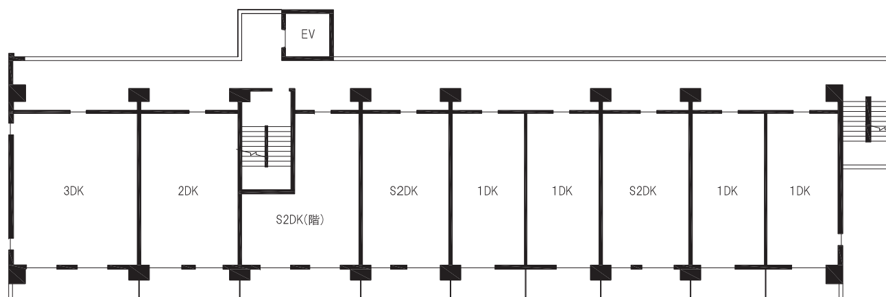
3～8階平面図
