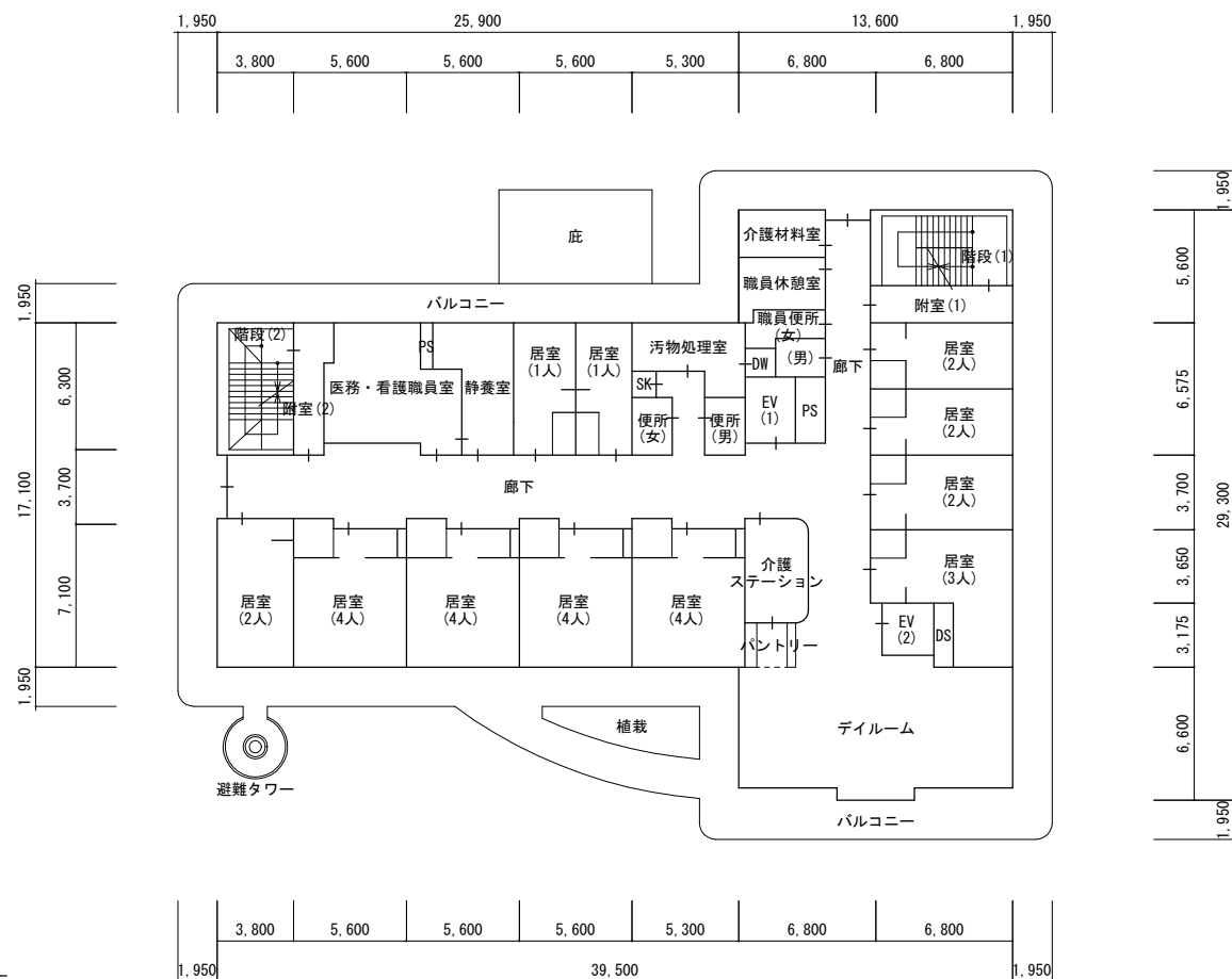
2階平面図 S=1/400
