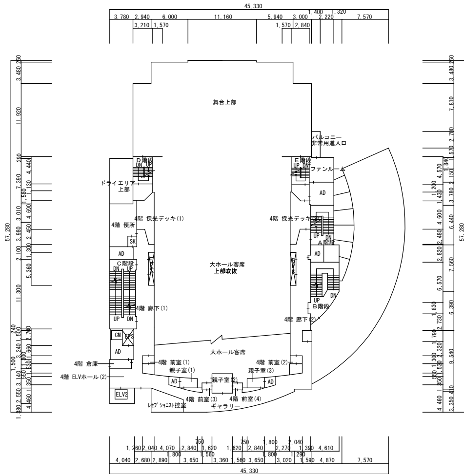
4階平面図 S=1/600 (江東公会堂)
