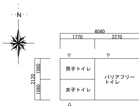
平面図 S=1/100 (猿江恩賜公園公衆便所)
