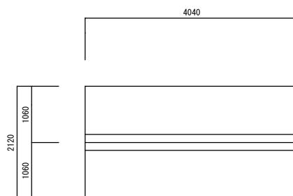
屋根伏図 S=1/100 (猿江恩賜公園公衆便所)
