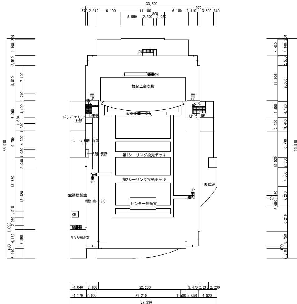
5階平面図 S=1/600 (江東公会堂)
