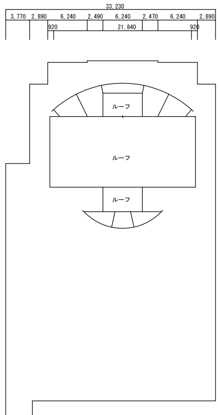
塔屋伏図1 S=1/600 (江東公会堂)
