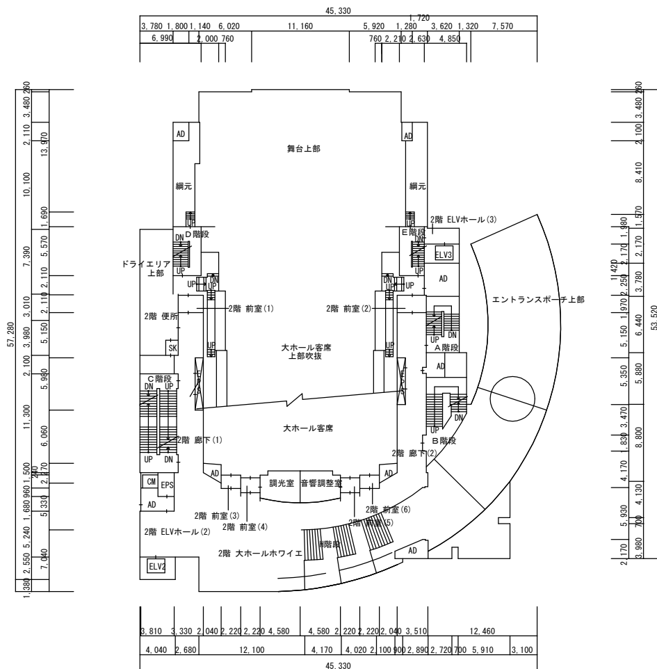
2階平面図 S=1/600 (江東公会堂)
