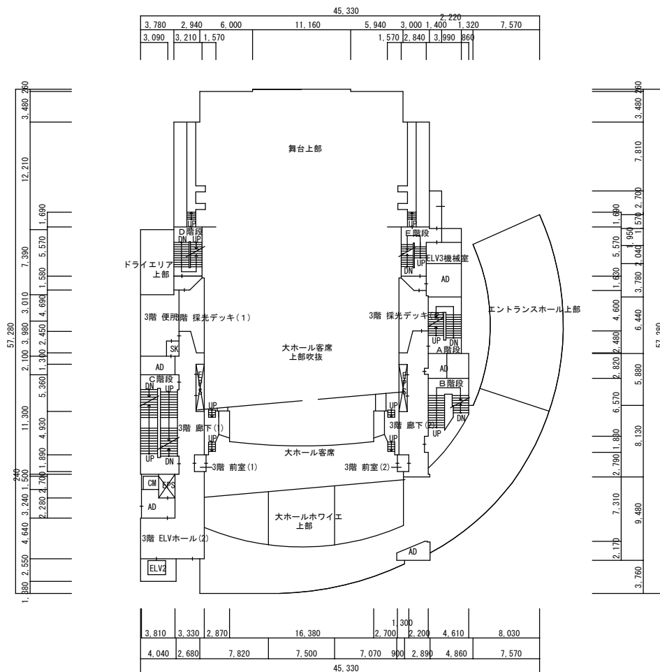
3階平面図 S=1/600 (江東公会堂)
