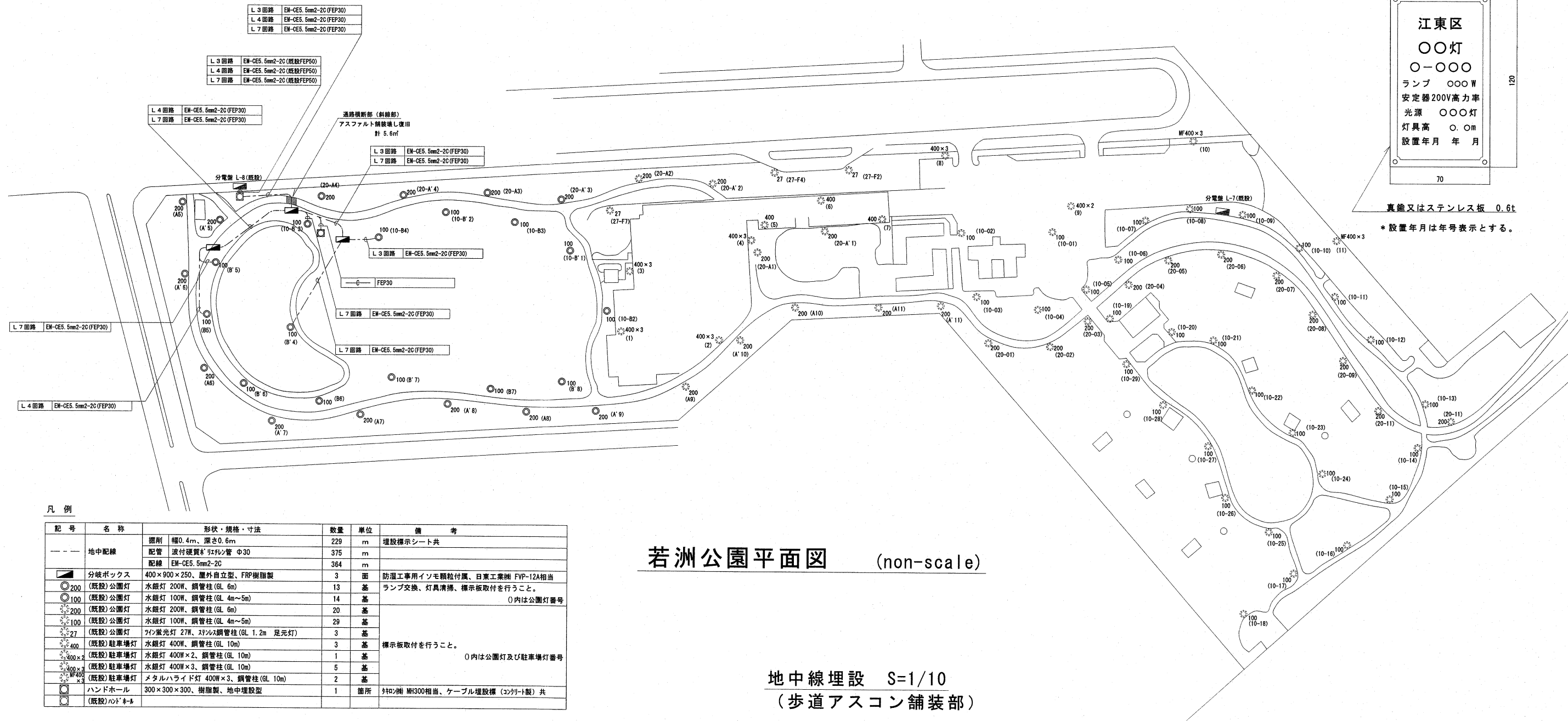
地中線埋設 S=1/10
