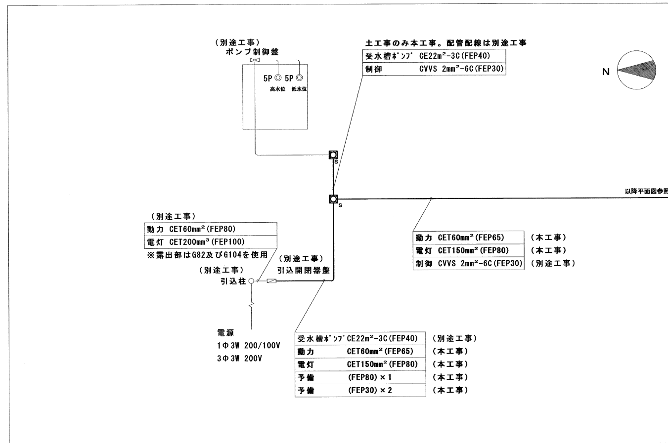
(電気) 詳細図 1 S=1:200
