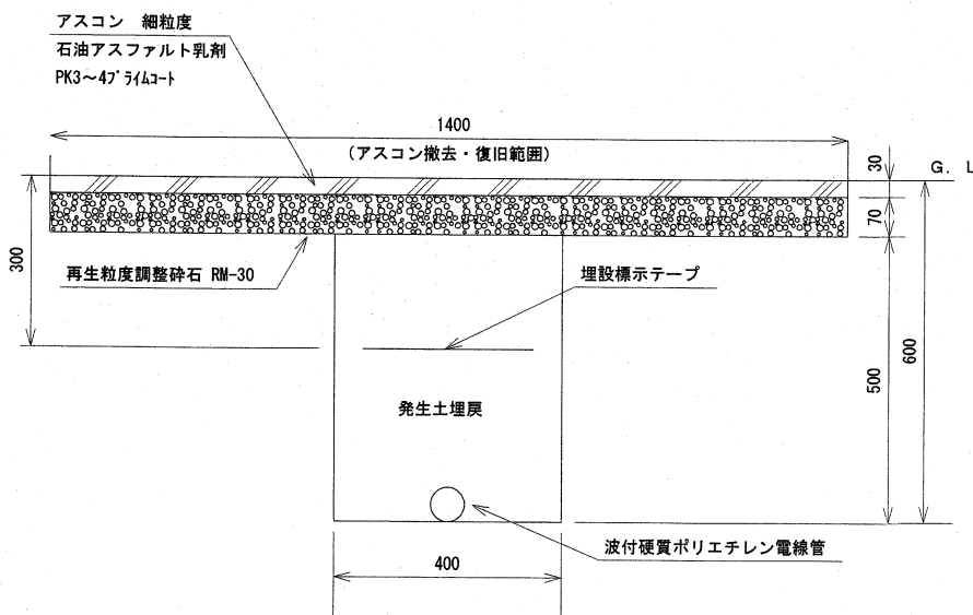
地中線埋設 S=1/10 (歩道アスコン舗装部)
