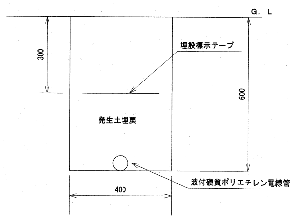
地中線埋設 S=1/10
