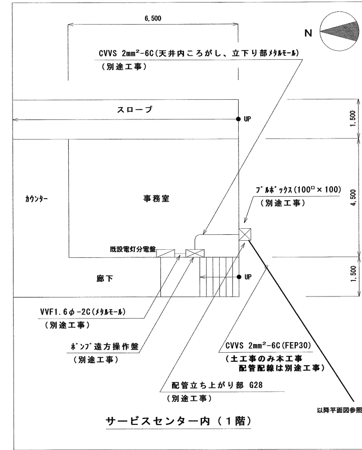
(電気) 詳細図 2 S=1:100
