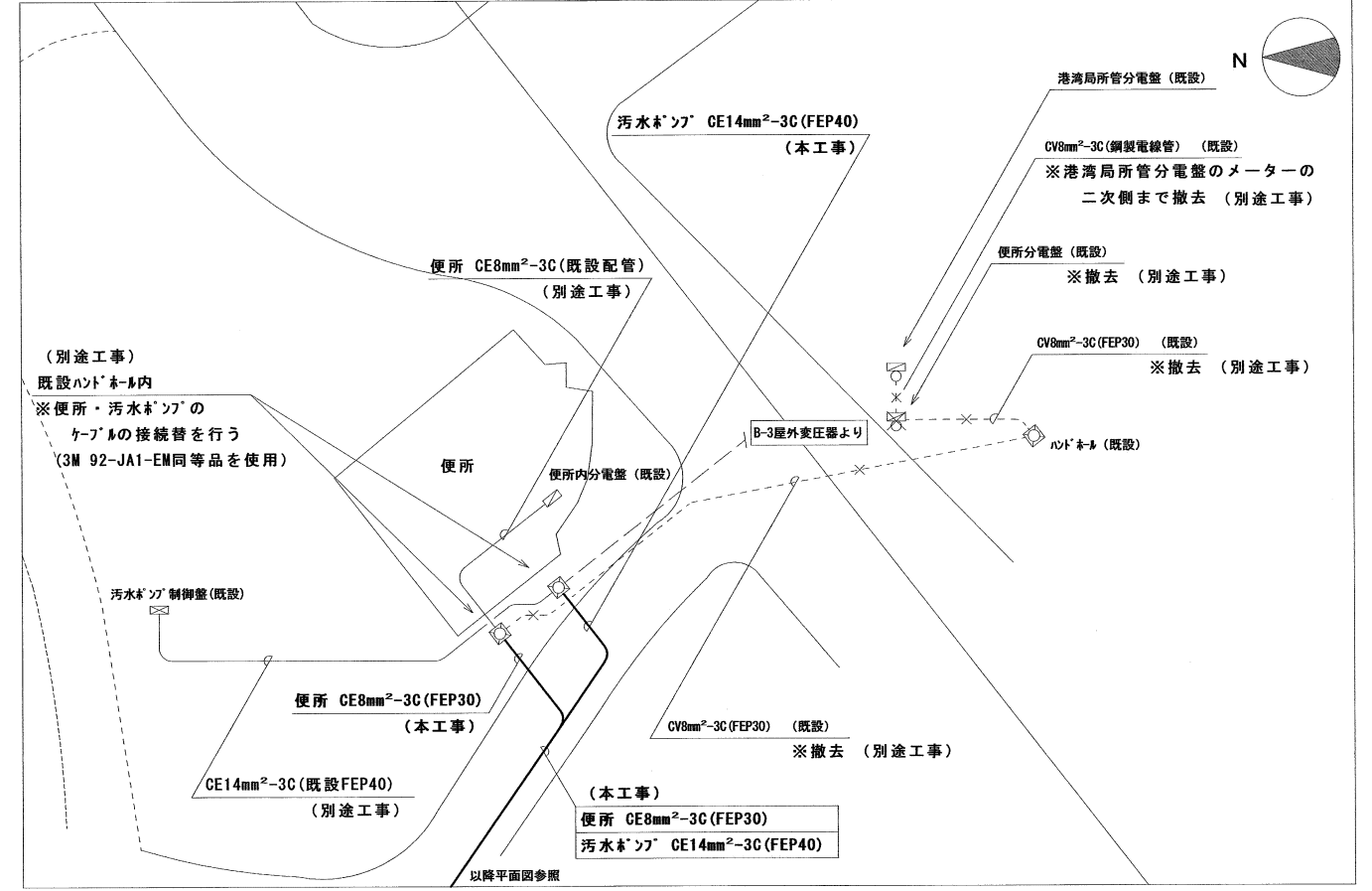
(電気) 詳細図 4 S=1:200
