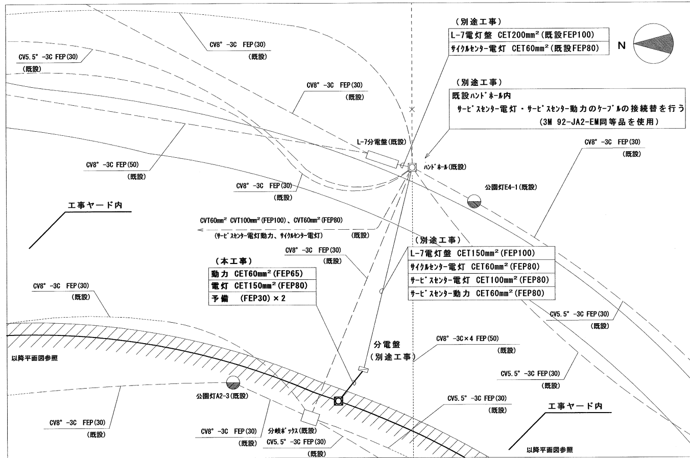
(電気) 詳細図 3 S=1:200
