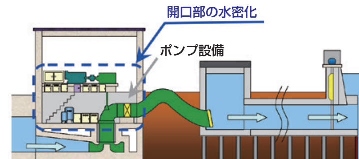
排水機場の耐水対策
