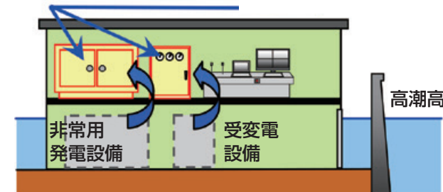
水門管理棟の耐水対策
