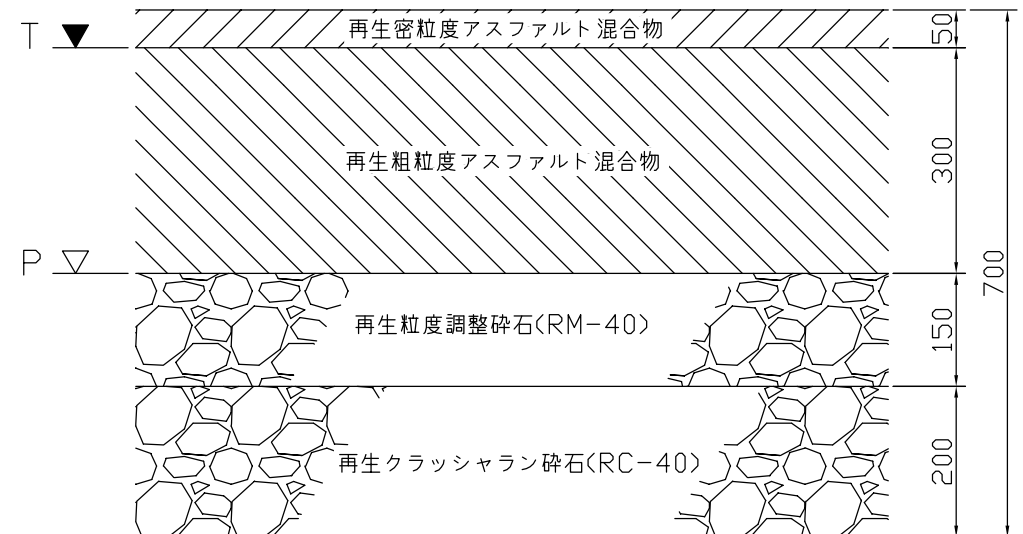
アスファルトコンクリート舗装70型
