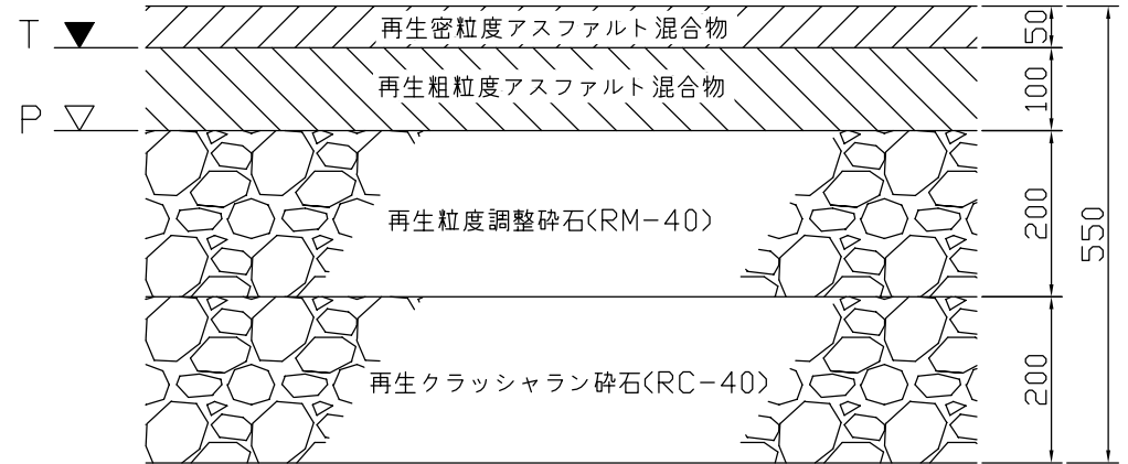
アスファルトコンクリート舗装70型
