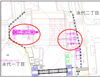
【図-1】 道路上に重機を配置して施工
