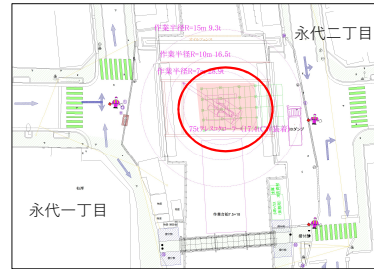
【図-2】 河川上にステージ構築し、重機を配置して施工
