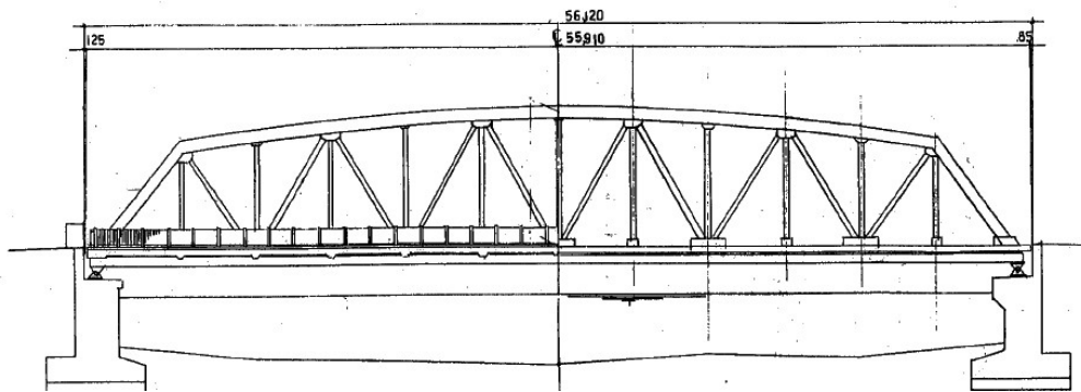
景観整備工事時の一般図
