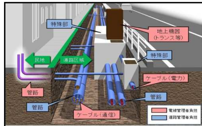
【標準断面図】
