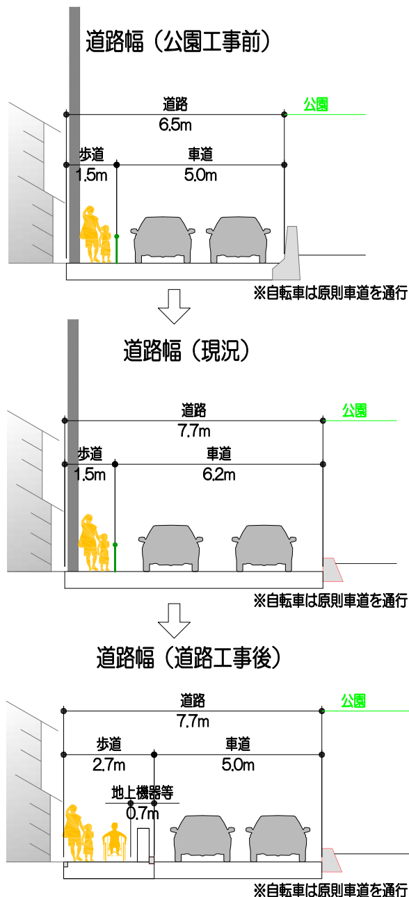
〈標準横断図〉
