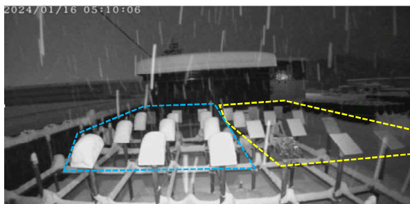
《着雪を検証した実験》
