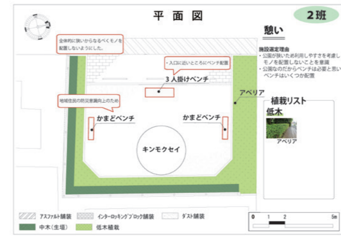
図2 2班の平面図案
