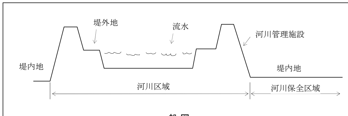
一般図
