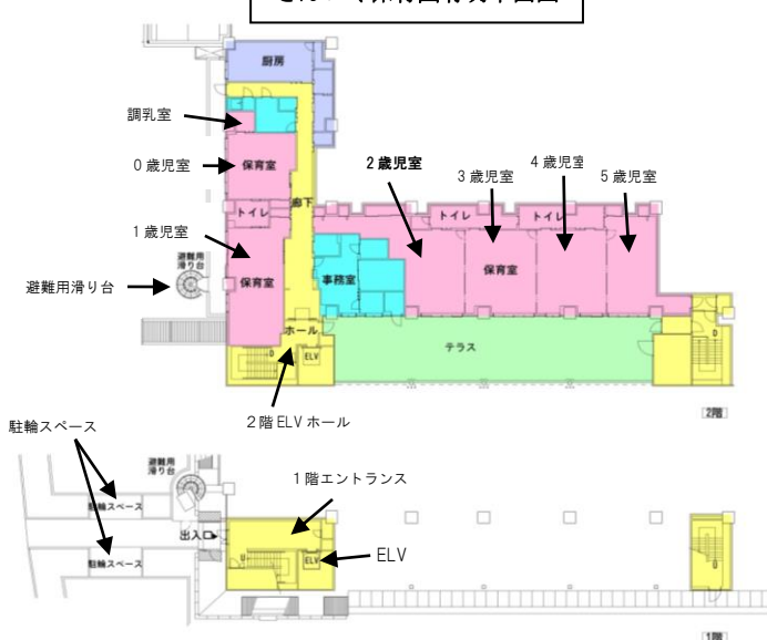
さんいく保育園有明平面図
