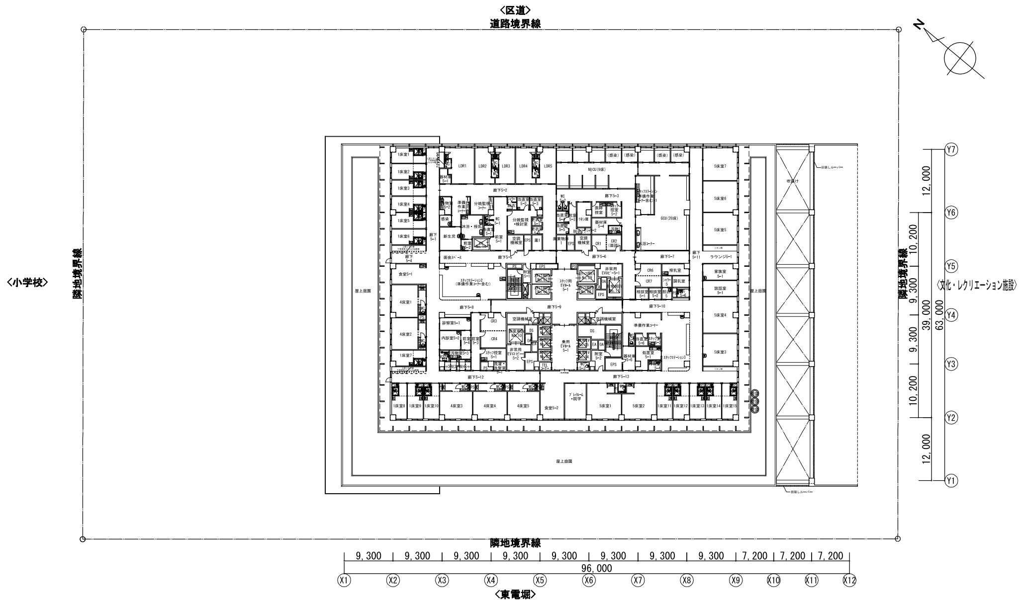
5階平面図
