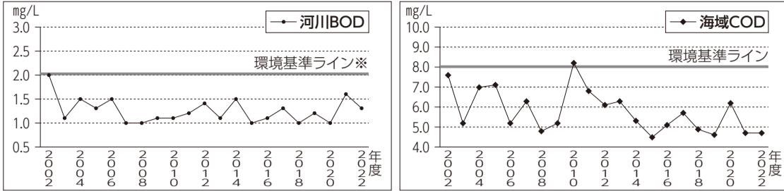
河川BODと海域CODの経年変化(区内平均値)
