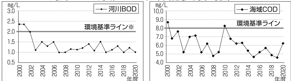
河川BODと海域CODの経年変化(区内平均値)
