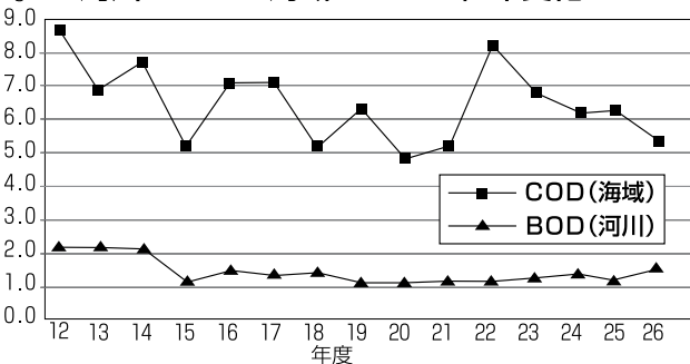
mg/L 河川BODと海域CODの経年変化
