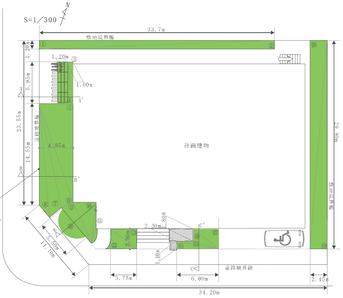
緑化面積求積図
