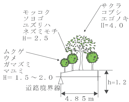
B-B' 断面図
