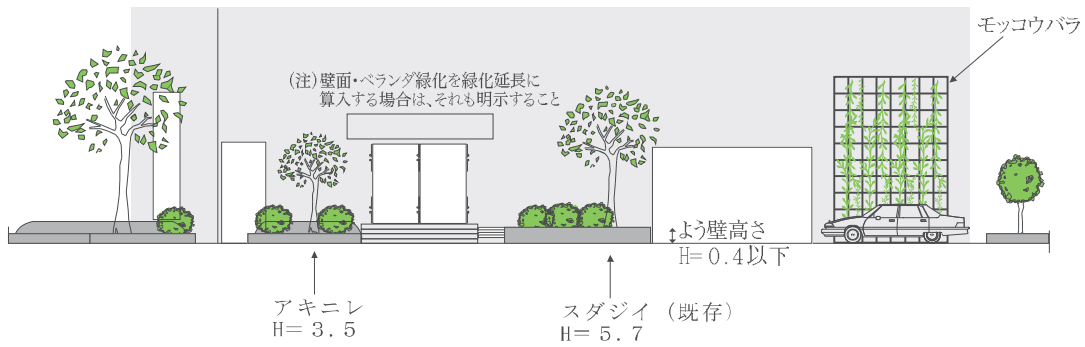
接道部立面図（南側）
