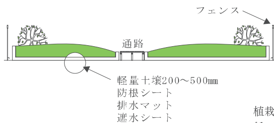
D-D' 断面図
