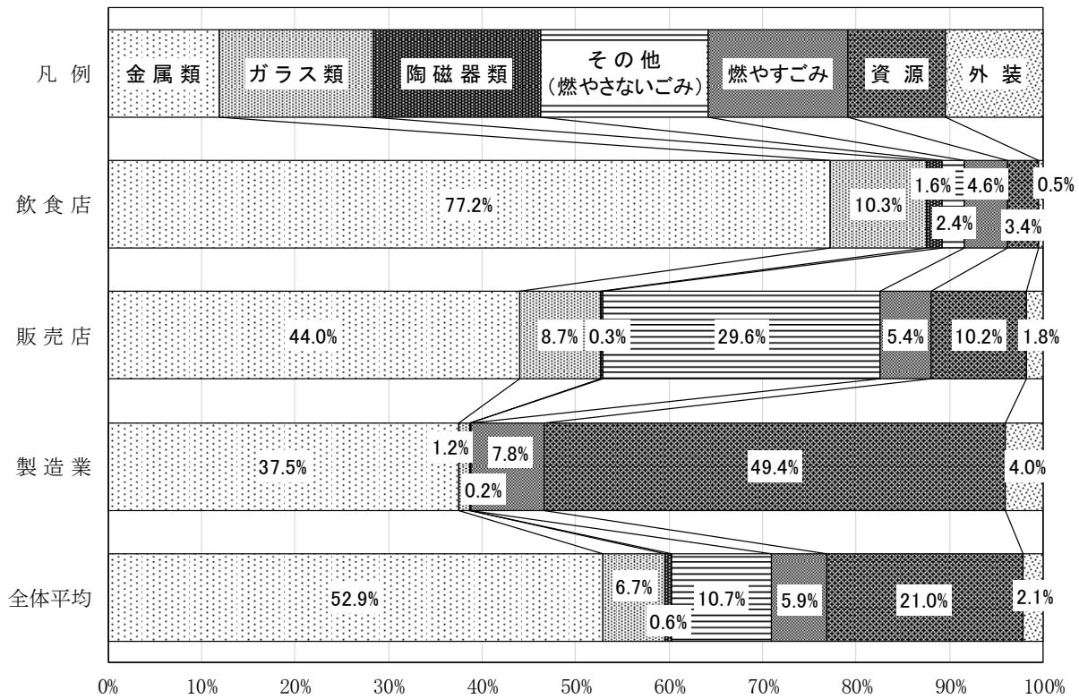
図 1-14 事業系ごみの燃やさないごみの組成割合（業種別）
